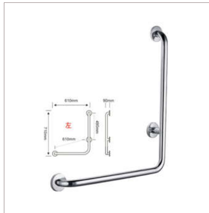
GB12 90° Left 50*70*9cm 60*70*9cm 70*70*9cm
